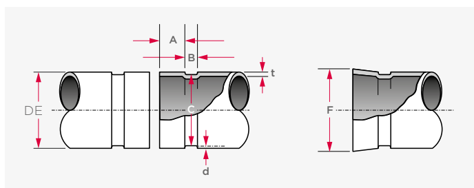
dimensions standard du rouleau et de la rainure
