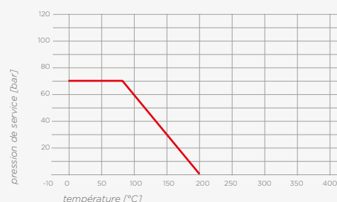
plage de pression-température
