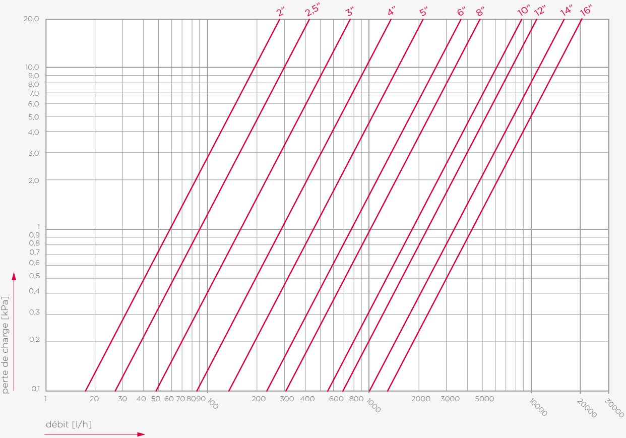
plage de débit
