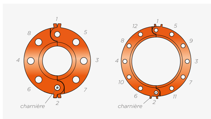
boulons 7043 (classe ANSI 300)
